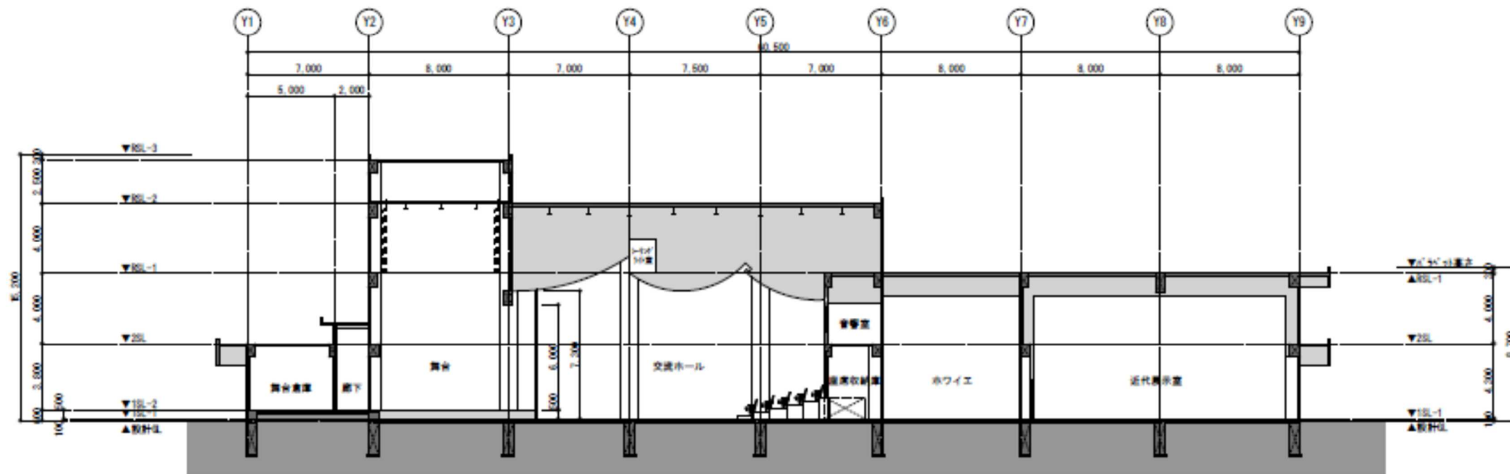
( 断面图 )
