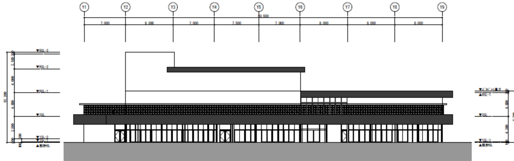
( 立面图 )
