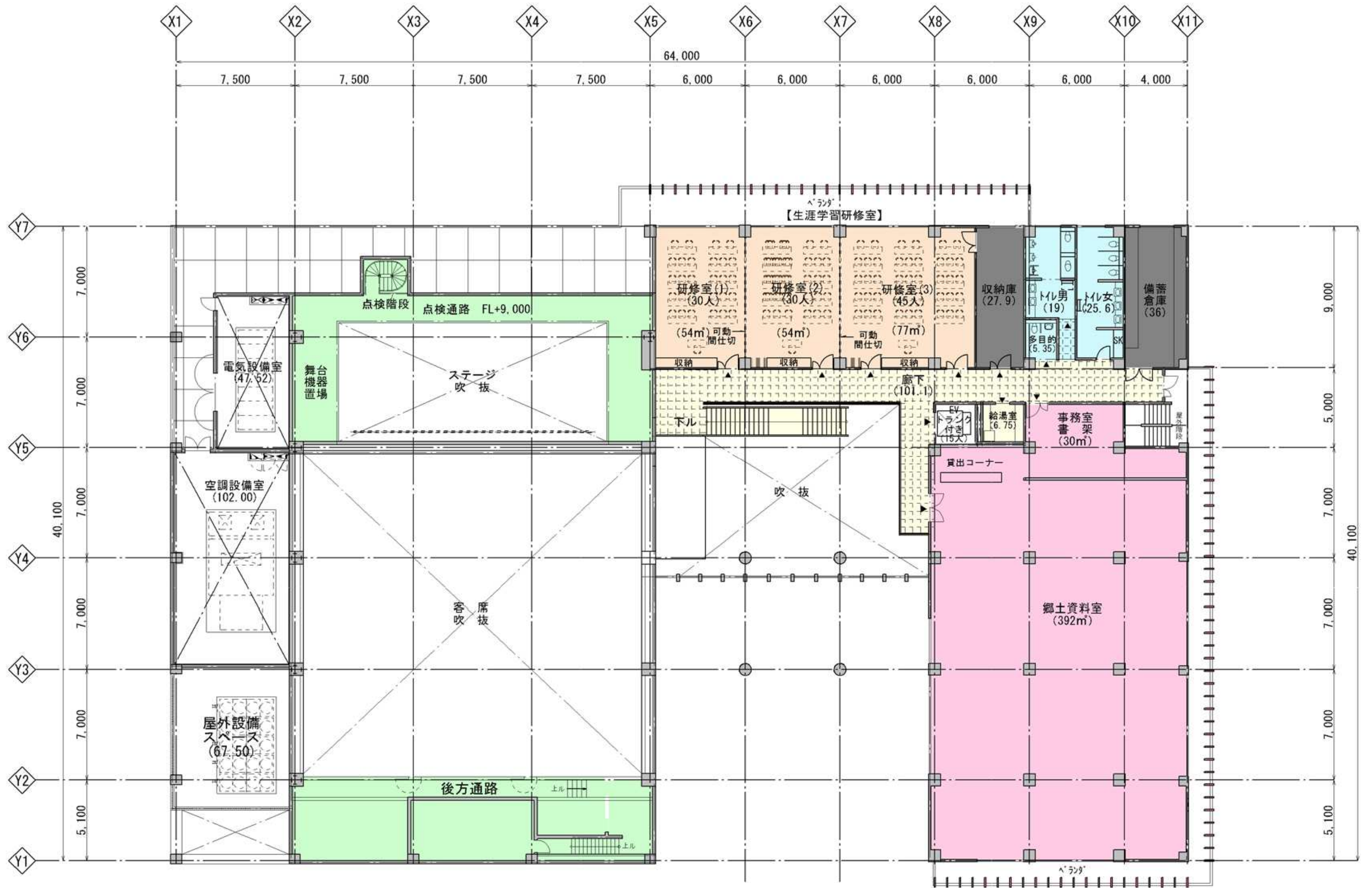
<2階平面図>
